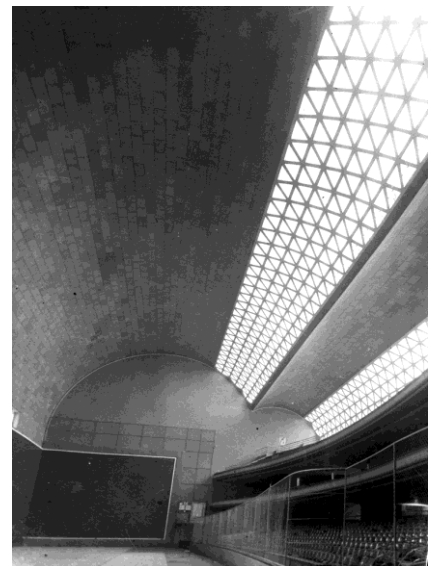
Figura 11: Mercado de Algeciras Market, Hipódromo de la Zarzuela y Frontón Recoletos de Madrid
