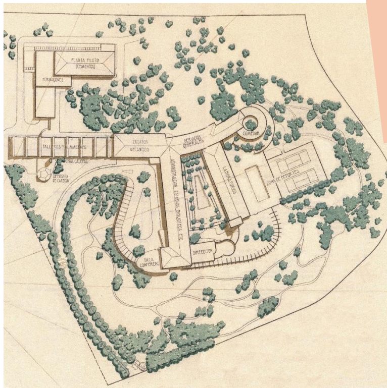
Figura 1. Planta del Edificio del Instituto Eduardo Torroja 1953
