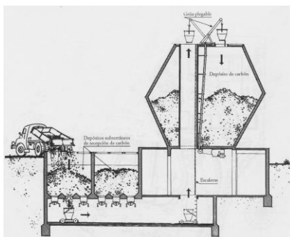
Figura 3. Dodecaedro. Silo de carbón
