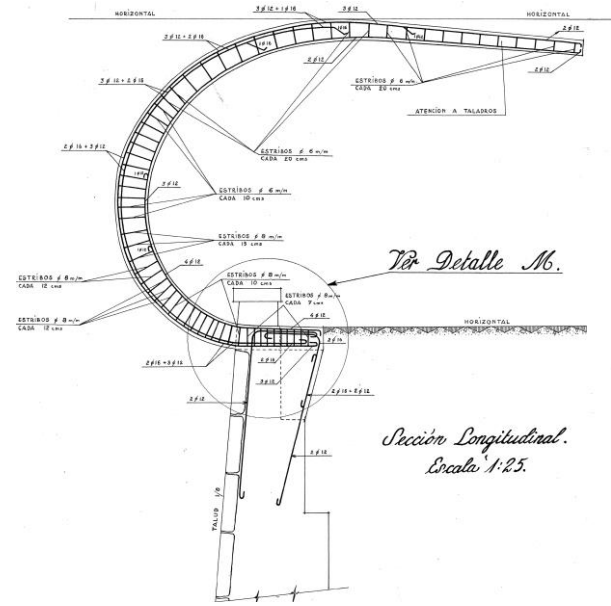
Figura 9. Pérgola de hormigón armado en voladizo
